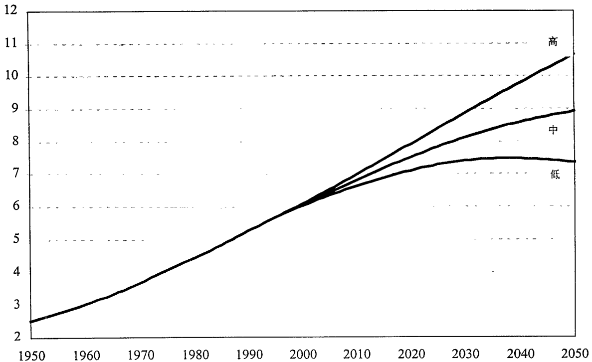
图一. 1950-2050 年世界人口规模:过去估计数和中、高、低生育率变量 (10 亿)
