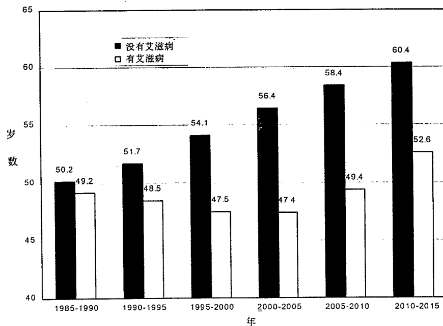
图三. 1985-1990 年至 2010-2015 年,29 个非洲国家有或无艾滋病情况下的出生时预期寿命
